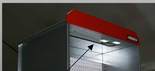
Indbygget lysstofarmatur for korrekt arbejdsbelysning
